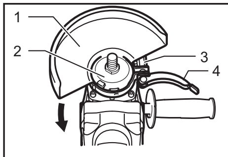
► 1. Carter de meule 2. Cage de roulement 3. Écrou 4. Levier
