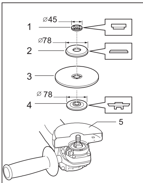
► 1. Contre-écrou 2. Flasque extérieur 78 3. Meule abrasive à tronçonner / roue diamantée 4. Bague interne 78 5. Carter de meule pour meule abrasive à tronçonner / roue diamantée
