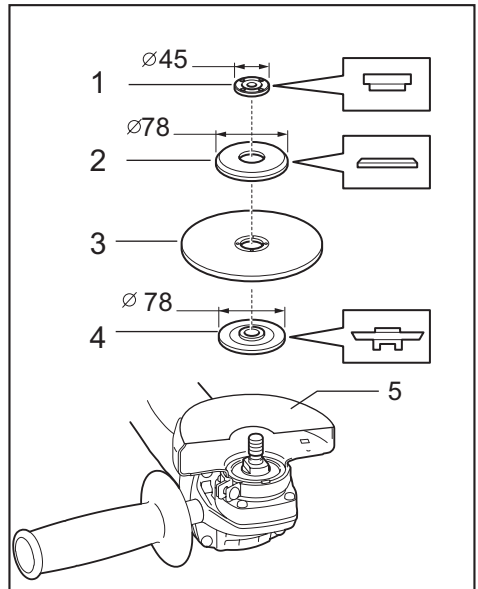
► 1. Contratuercas 2. Brida exterior 78 3. Disco de corte abrasivo / Disco de diamante 4. Brida interior 78 5. Protector de disco para disco de corte abrasivo / disco de diamante
